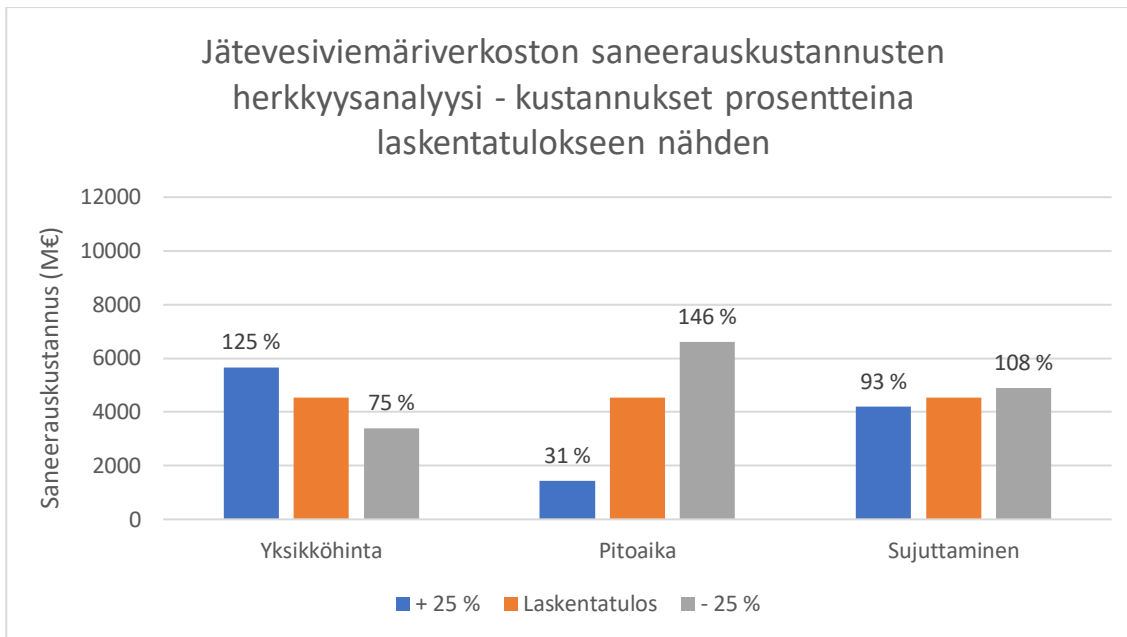
Kuva 19. Herkkyysanalyysin tulokset–jätevesiviemäriverkosto.
