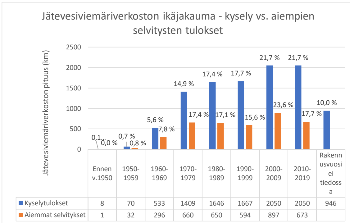
Kuva 13. Jätevesiviemäriverkoston keskimääräinen ikäjakauma kyselytulosten ja AFRY Finland Oy:n konsulttitöiden perusteella (HSY ei mukana).
