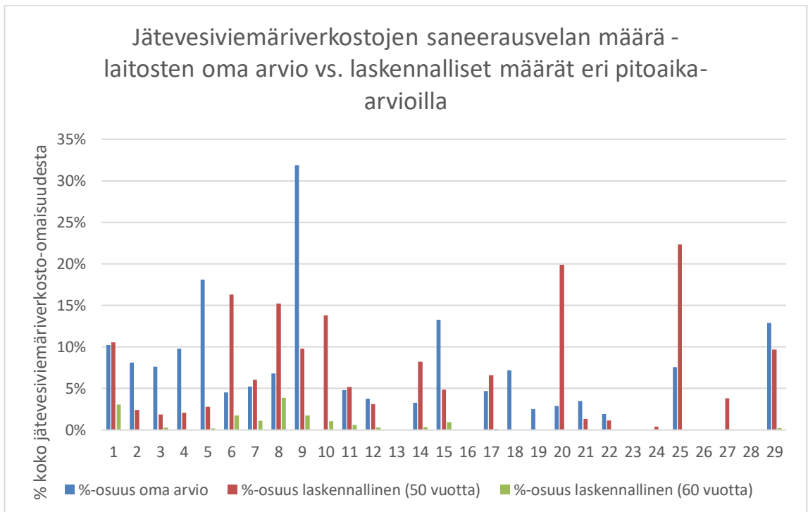
Kuva 21. Jätevesiviemäriverkostojen saneerausvelan määrä laitosten omien arvioiden ja pitoaikaoletuksien mukaan.
