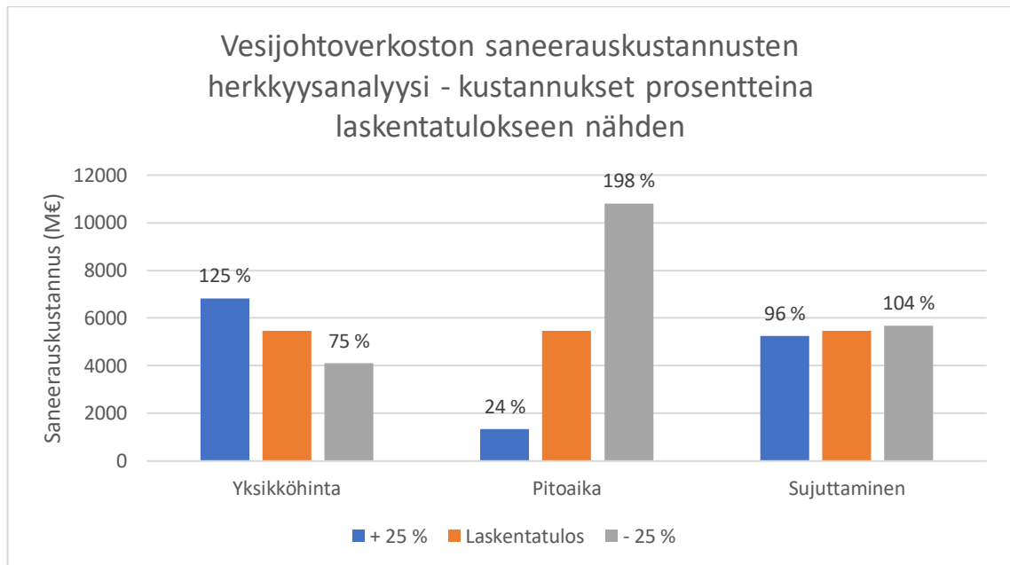
Kuva 18. Herkkyyshanalyysin tulokset–vesijohtoverkosto.
