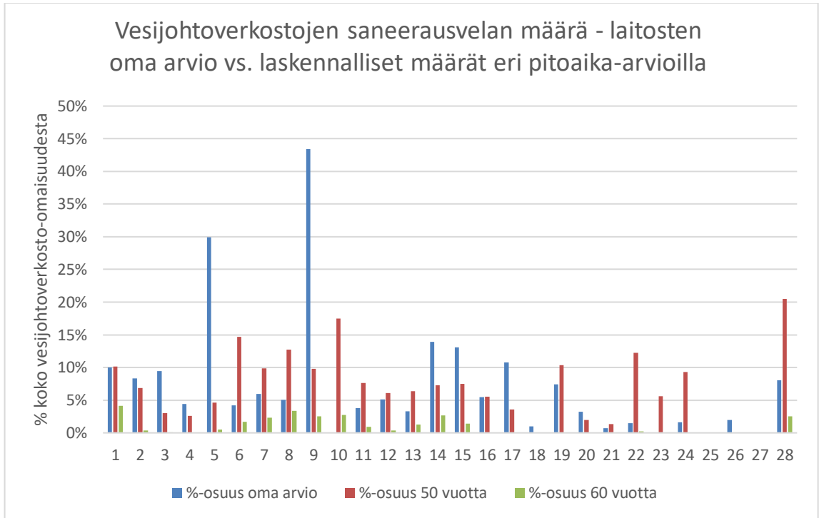
Kuva 20. Vesijohtoverkostojen saneerausvelan määrä laitosten omien arvioiden ja pitoaikaoletuksien mukaan.
