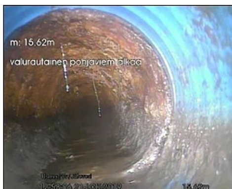
100 mm valurauta alkaa, vähäinen pinta- vaurio, klo 0-12
