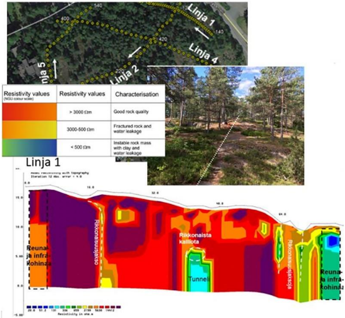
Kuva 24. Esimerkki sähköisen tomografiakuvauksen tuloksista Espoon Piispankallion itäpuolen kallioalueella olevan viemäritunnelin ympäriltä. Tuloksilla voidaan osoittaa kallion eheyttä ja laatua sekä rikkonaisuusjaksojen sijaintia.
