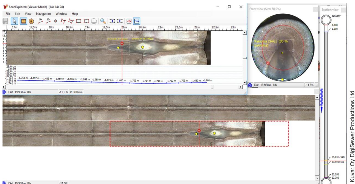
Kuva 16. Esimerkki Digikuvauksella saatavasta kaivovälikohtaisesta datasta. Kuvassa on demonstroitu painuman havainnointia, joka näkyy etukuvassa lammikkona ja avattussa kuvassa vedenpinnan leventymisenä sekä viettokaltevuuskäyrässä.
