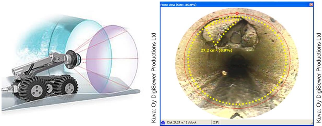
Kuva 19. Digikamera varustettuna laserpisteitä lähettävällä laser-renkaalla ja esimerkki mittaamisesta.
