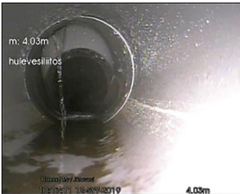
110 mm muovi, liittymä, tonttviemäriin liittyy tonttihulevesiviemäri klo 11
