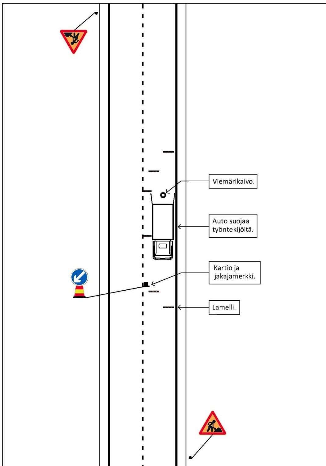
Kuva 1. Esimerkki lyhytkestoisen työn liikenteenohjaussuunnitelmasta.
