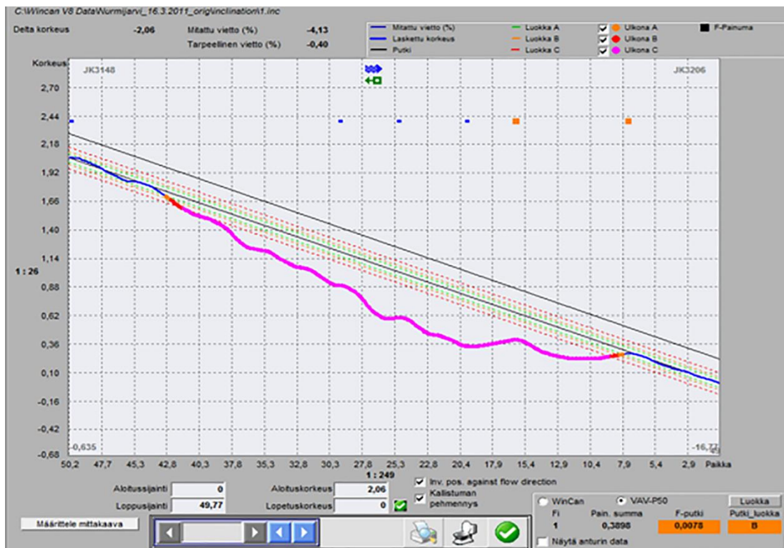
Kuva 17. Esimerkki viettokaltevuusmittauksen tuloksesta.
