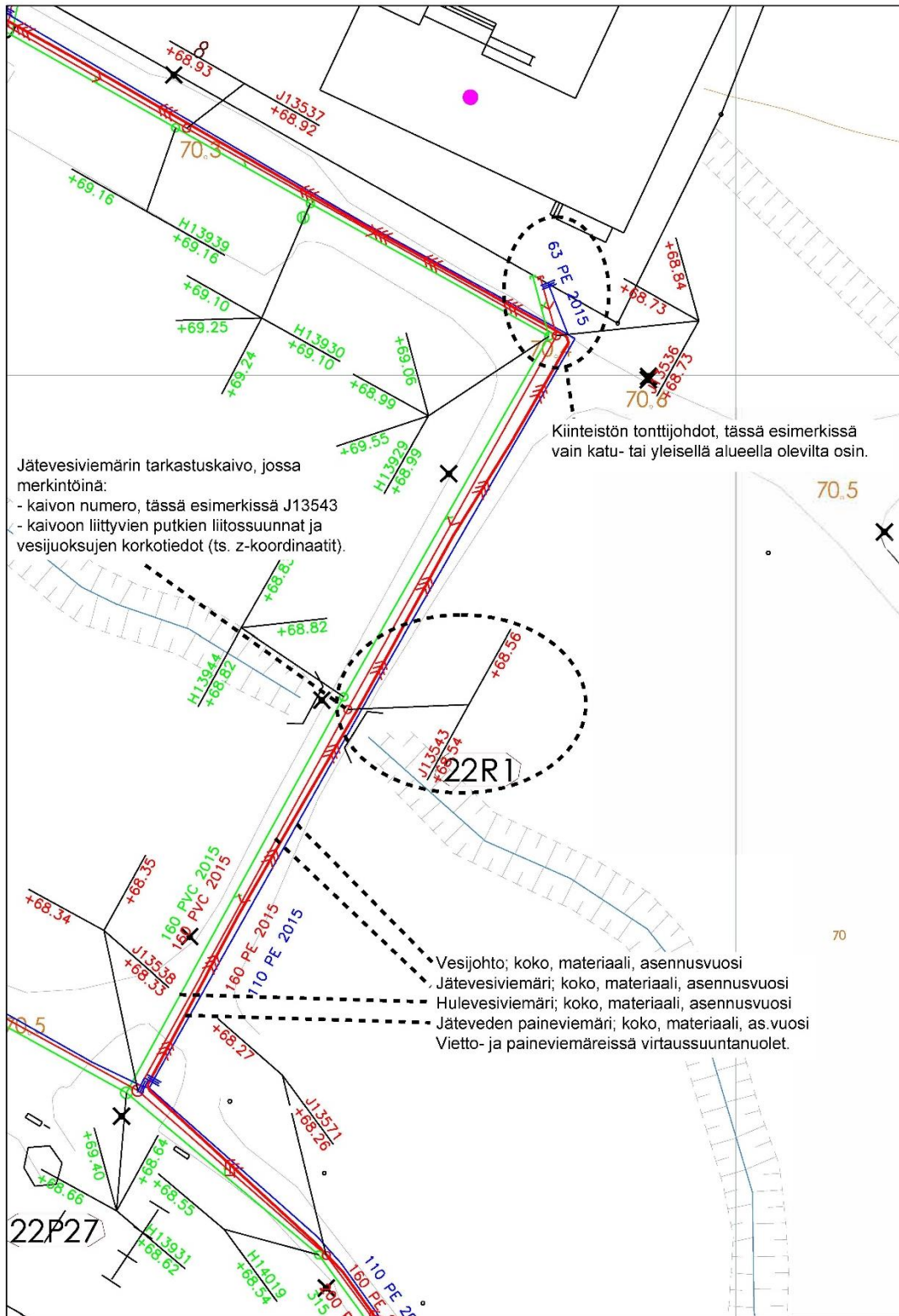
Kuva 3. Esimerkki verkostokartasta. (Kuva: Aqua Palvelu Oy)
