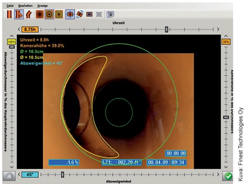
Kuva 21. Liittyvän putken halkaisijan mittaaminen kuvatusta videosta.
