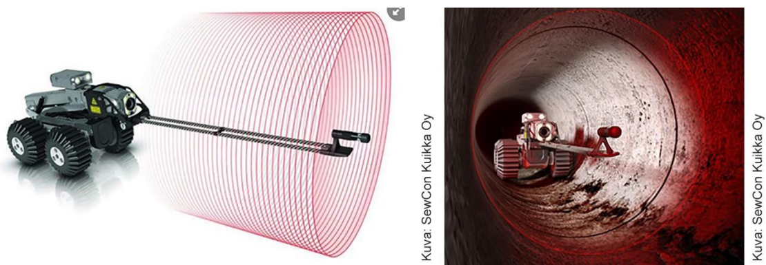
Kuva 18. Lasermittatikulla varustettu läpiajettava kamera.
