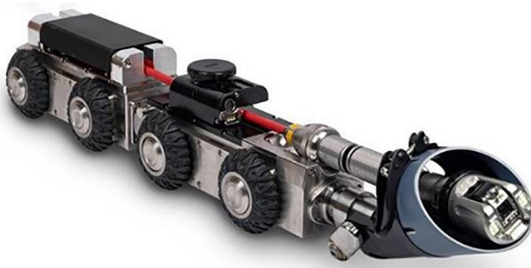
Kuva 14. Esimerkki satelliittikameralla varustetusta läpiajettavasta kamerasta.
