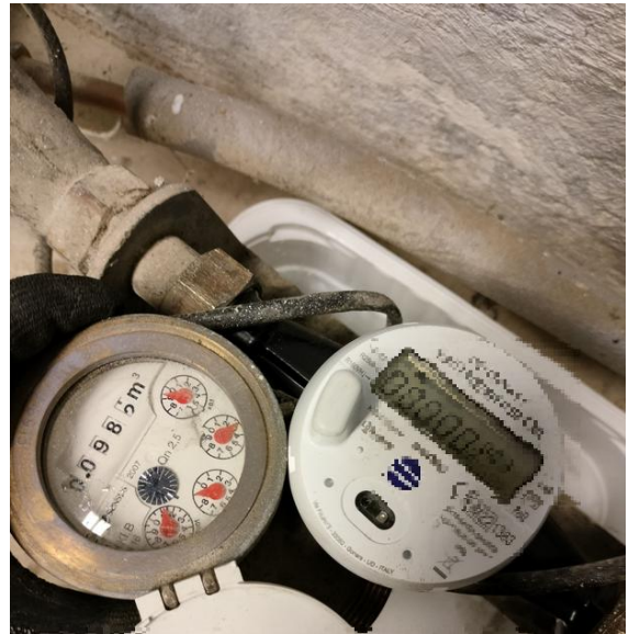
Kuva 15. Etäluettava vesimittari asennettuna vanhan mekaanisen mittarin tilalle. Turun Vesihuolto Oy.
